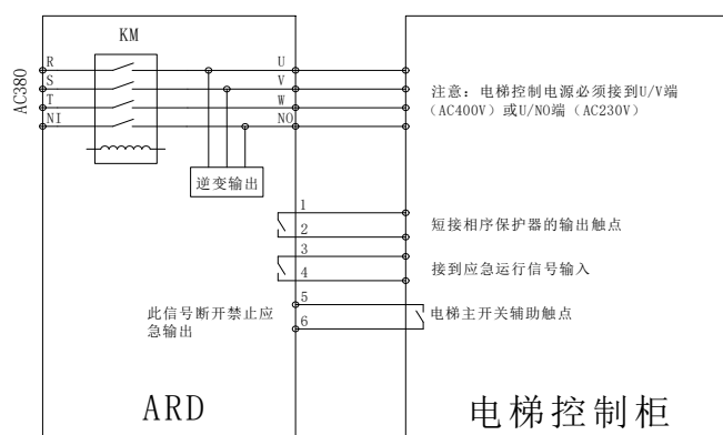
三相典型连接示意图
